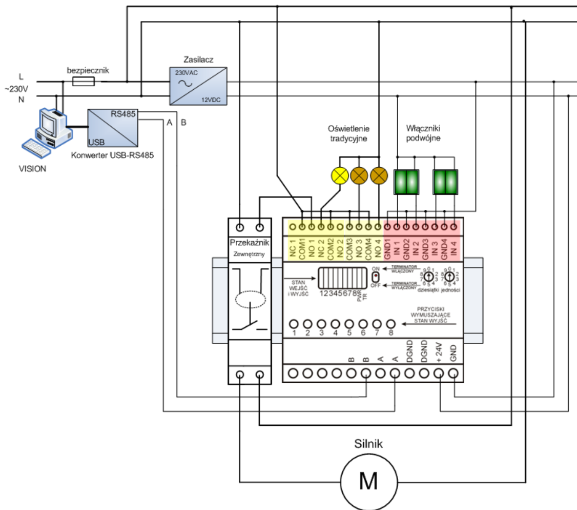
Rys. 12. Schemat aplikacji nr 2
