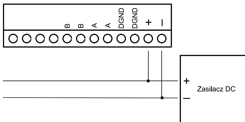
Rys. 10. Schemat podłączenia urządzenia do napięcia zasilania
