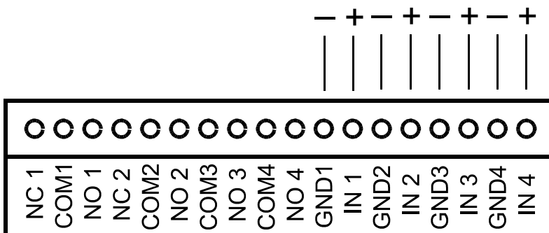
Rysunek 6. Schemat podłączeń wejść cyfrowych
