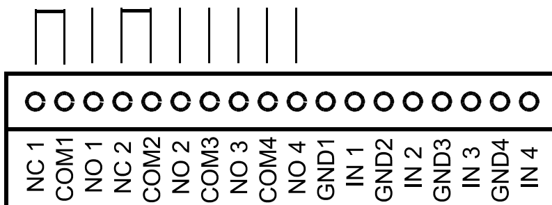
Rys. 7. Schemat połączeń wyjść przekaźnikowych podczas braku wysterowania przekaźników
