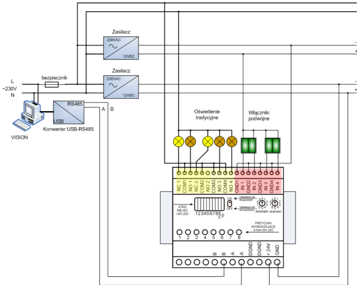
Rys. 11. Schemat aplikacji nr 1
