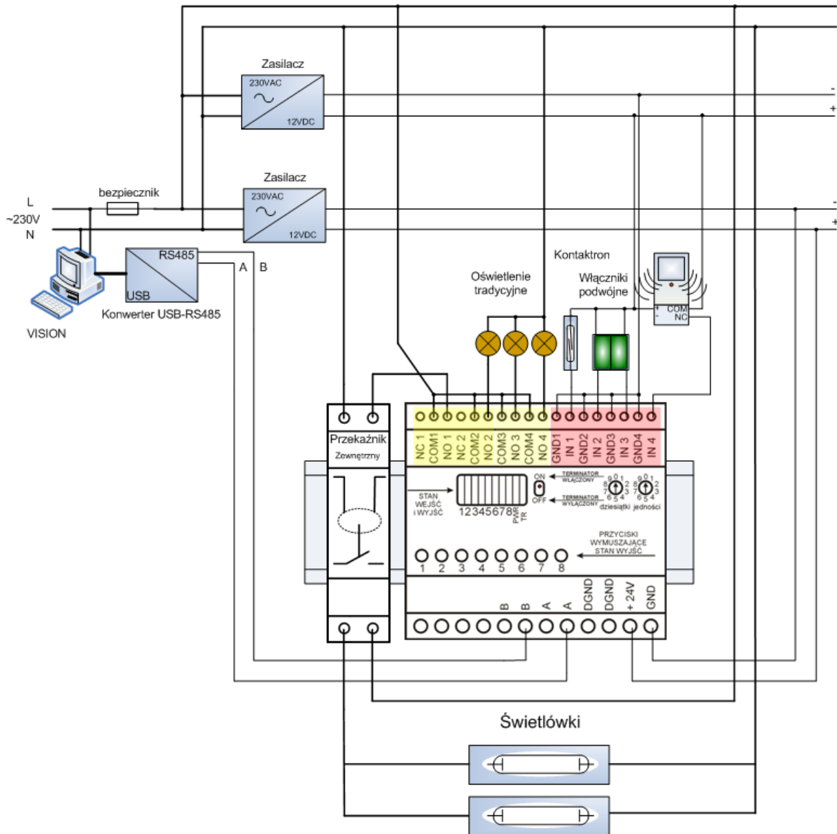
Rysunek 13. Schemat aplikacji nr 3
