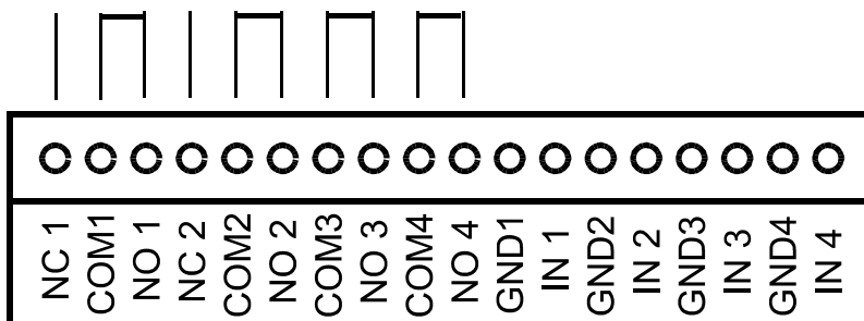
Rys. 8. Schemat połączeń wyjść przekaźnikowych podczas wysterowania przekaźników
